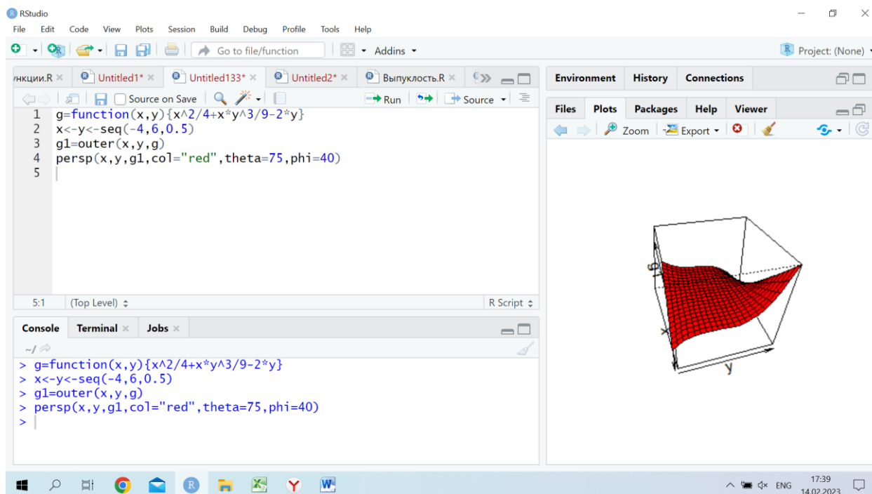
Рис.1 Код построения графика функции g = \frac{x^2}{4} + x \cdot \frac{y^3}{9} - 2y
